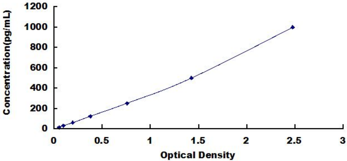
大鼠组织因子通道抑制因子(TFPI)检测试剂盒标准曲线
