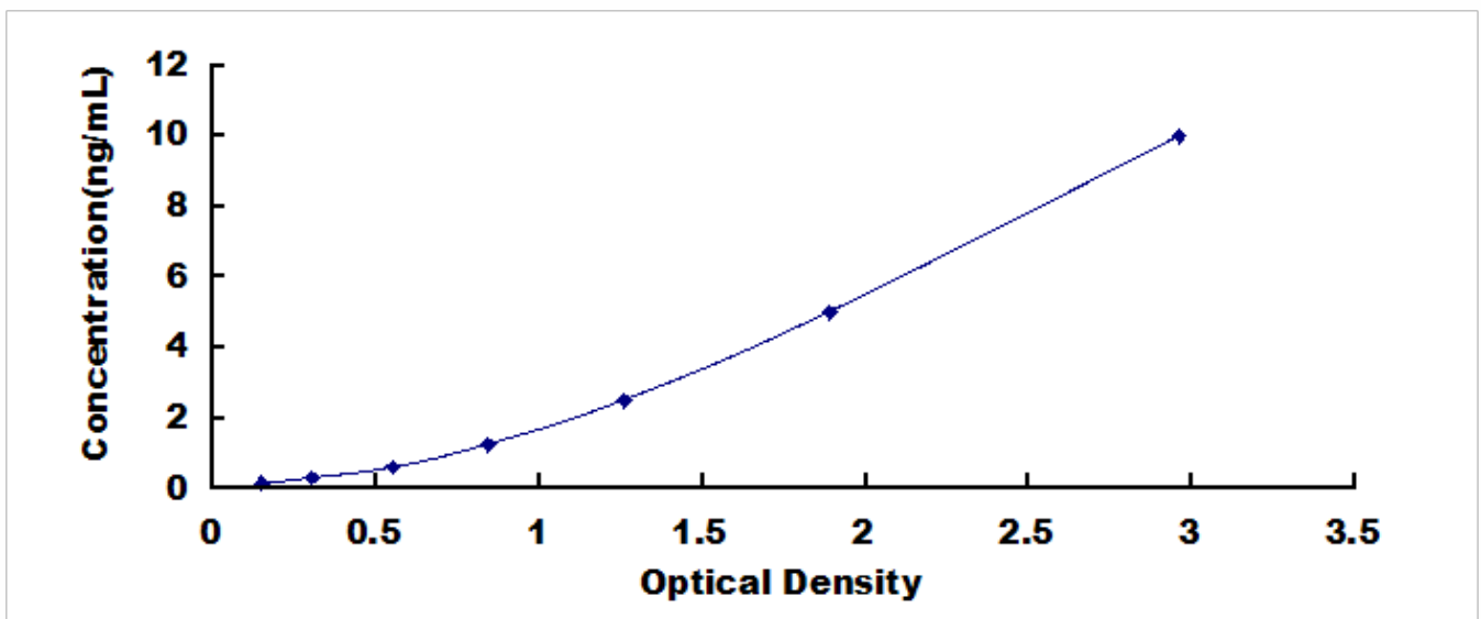
酪氨酸 3/色氨酸 5 单加氧酶活化蛋白 \theta (YWHA \theta ) 检测试剂盒标准曲线
