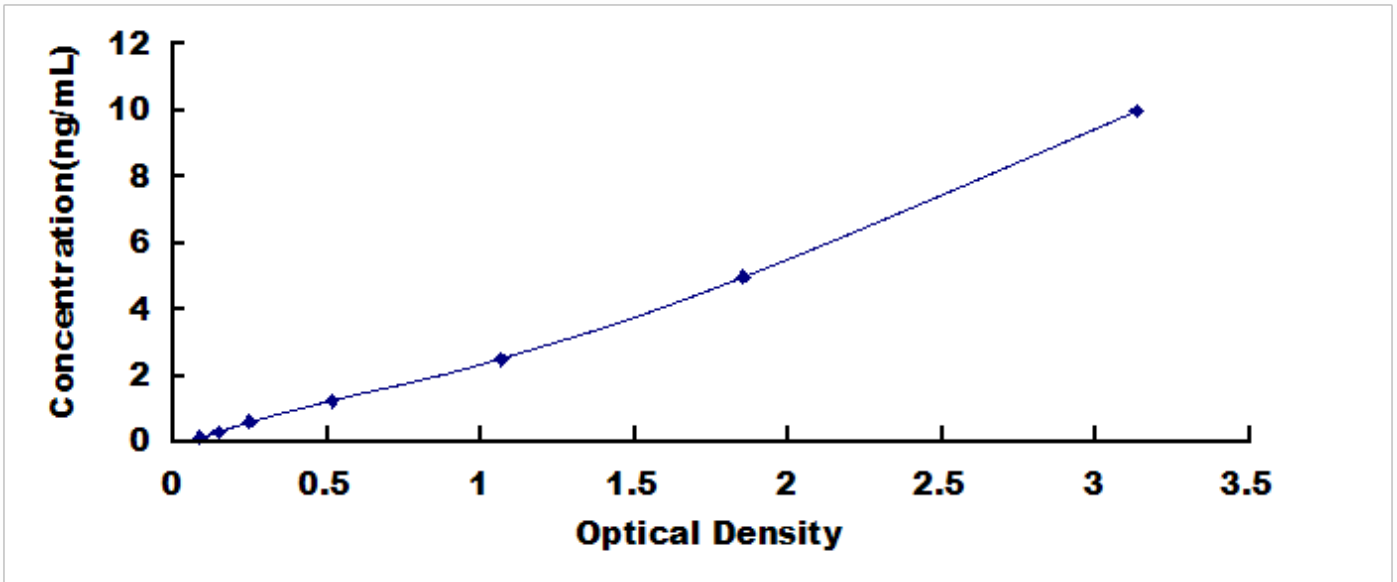
人 V-Erb B2 红白血病病毒癌基因同源物 3 (ErbB3) 检测试剂盒标准曲线
