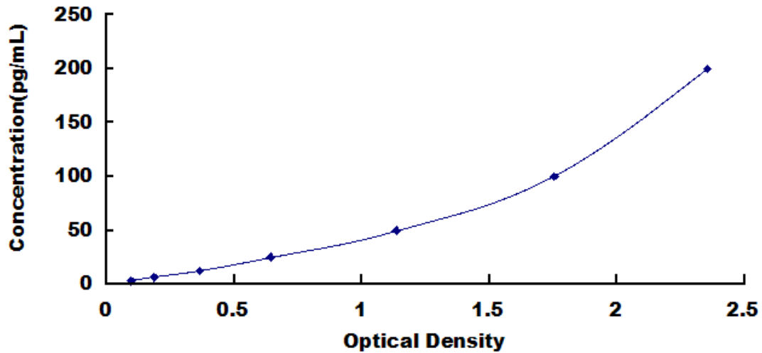
人 Adropin 蛋白 (AD) 检测试剂盒标准曲线
