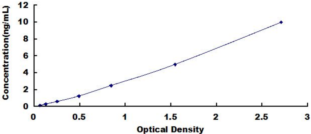
大鼠无翅型 MMTV 整合位点家族成员 3A (WNT3A) 检测试剂盒标准曲线
