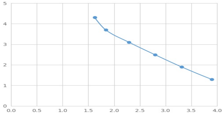
(17-羟孕酮)检测试剂盒标准曲线
