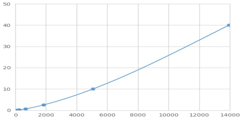
(5-甲基四氢叶酸高半胱氨酸甲基转移酶)检测试剂盒标准曲线
