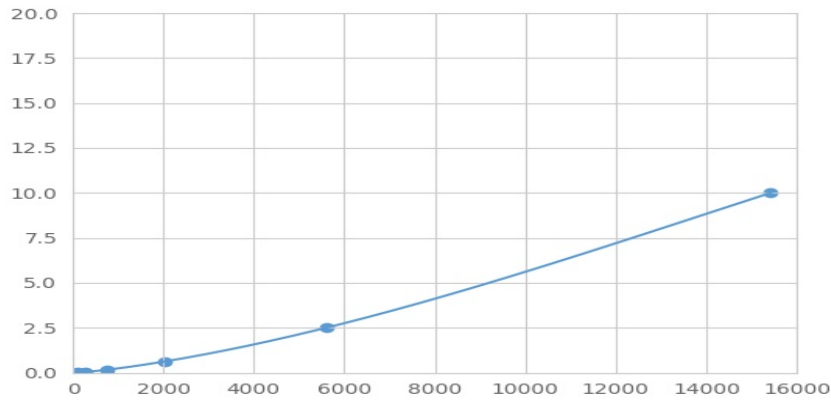
(ATP结合盒转运蛋白C12)检测试剂盒标准曲线
