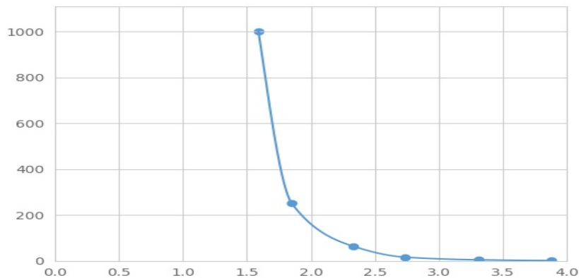
(乙酰胆碱)检测试剂盒标准曲线
