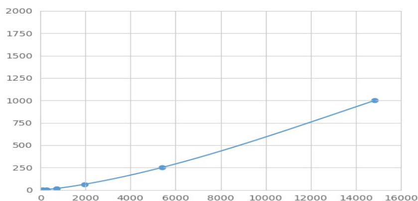
(铜蓝蛋白)检测试剂盒标准曲线
