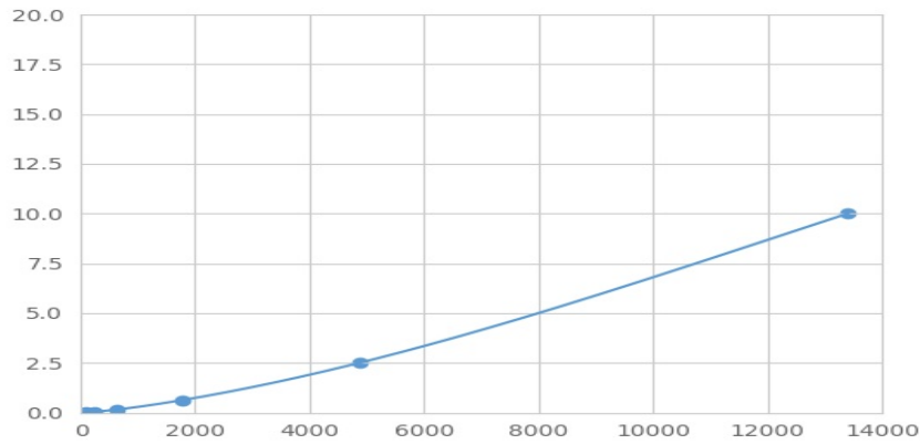
(封闭蛋白11)检测试剂盒标准曲线
