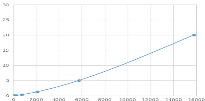
(细胞色素P450氧化还原酶)检测试剂盒标准曲线
