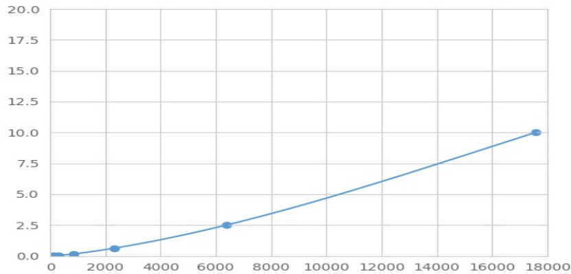
(角蛋白12)检测试剂盒标准曲线
