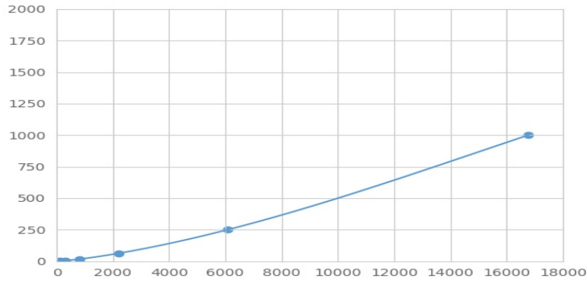
(细胞因子样蛋白1)检测试剂盒标准曲线
