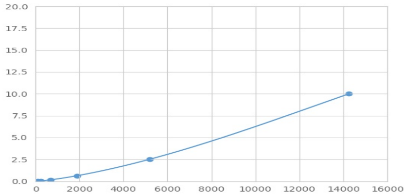
(EGF样域蛋白7)检测试剂盒标准曲线
