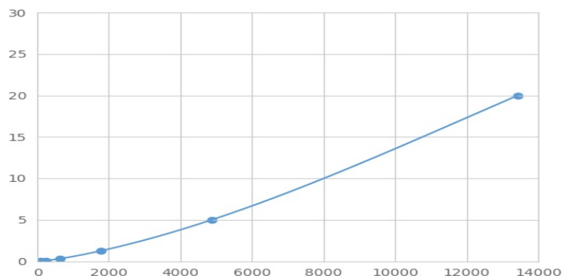
(齿状片段同源框蛋白2)检测试剂盒标准曲线
