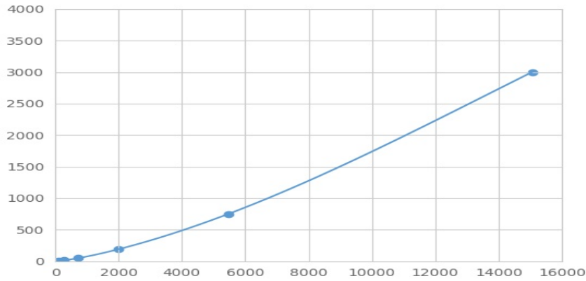
(细胞外信号调节激酶2)检测试剂盒标准曲线
