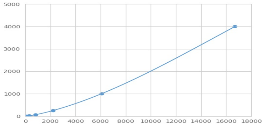
(法尼基二磷酸合酶)检测试剂盒标准曲线
