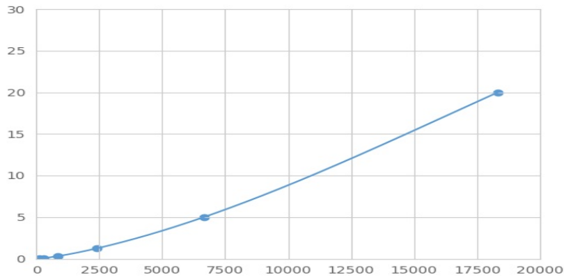
(岩藻糖苷酶 α L1)检测试剂盒标准曲线
