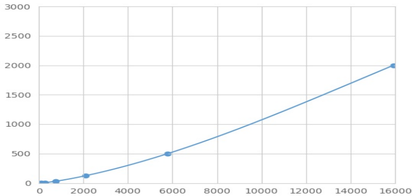
(葡萄糖脑苷脂酶)检测试剂盒标准曲线
