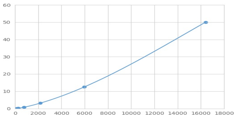
(糖基化磷脂酰肌醇特异性磷脂酶D1) 检测试剂盒标准曲线
