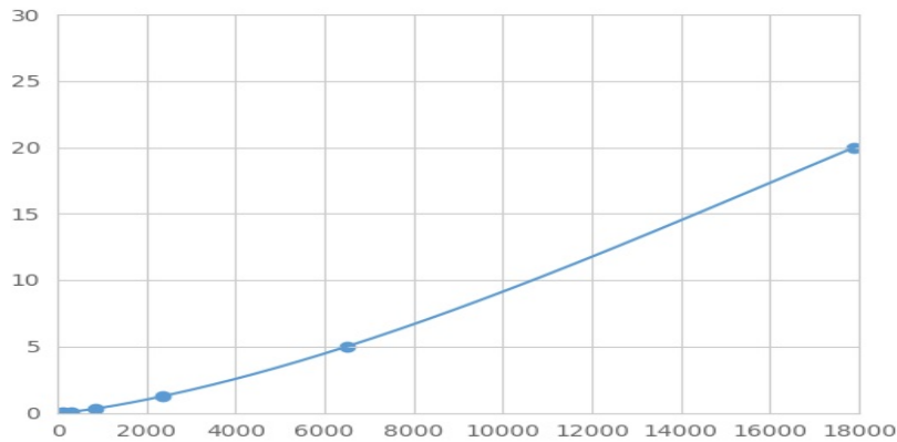
(高尔基体蛋白A8家族成员A)检测试剂盒标准曲线
