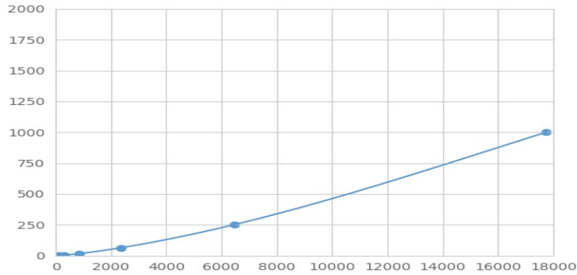
(抑制素 \alpha )检测试剂盒标准曲线
