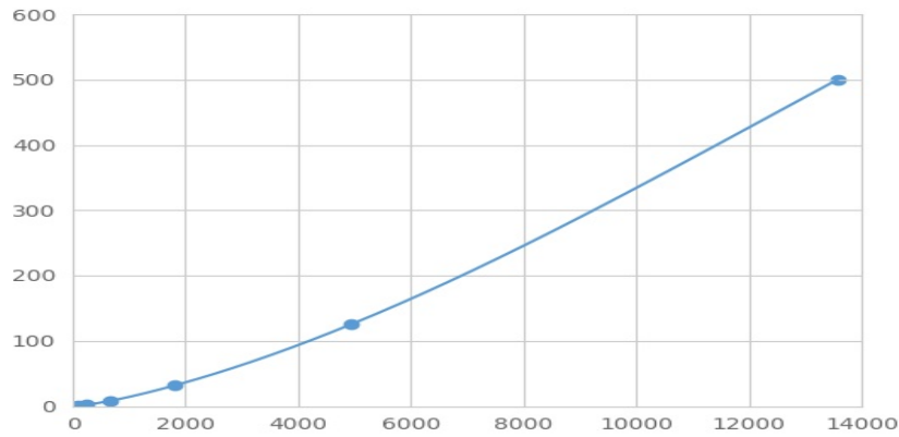
(白介素10)检测试剂盒标准曲线
