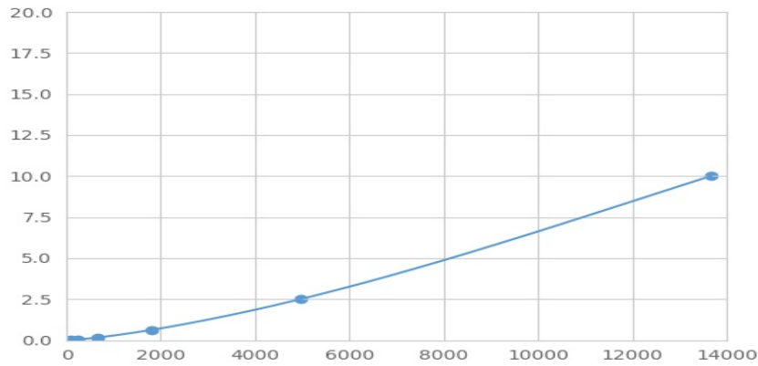
(激肽释放酶11)检测试剂盒标准曲线
