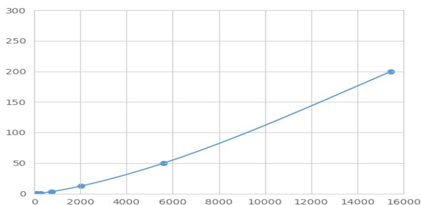
(内皮脂肪酶)检测试剂盒标准曲线
