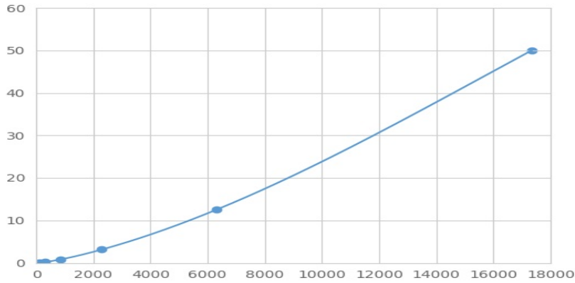
(苹果酸脱氢酶2) 检测试剂盒标准曲线
