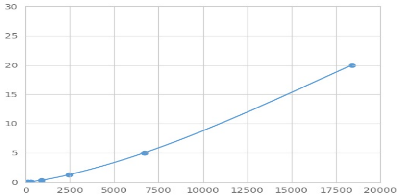
(金属硫蛋白1E)检测试剂盒标准曲线
