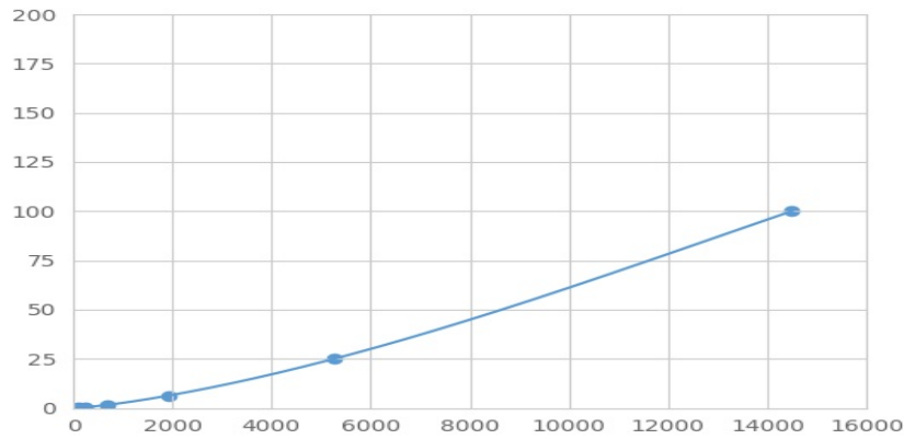
(甲羟戊酸脱羧酶)检测试剂盒标准曲线
