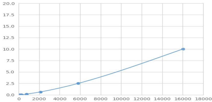
(脑红蛋白)检测试剂盒标准曲线
