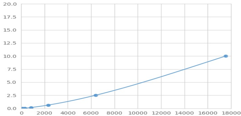
(中性鞘磷脂酶)检测试剂盒标准曲线
