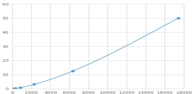
(巢蛋白)检测试剂盒标准曲线
