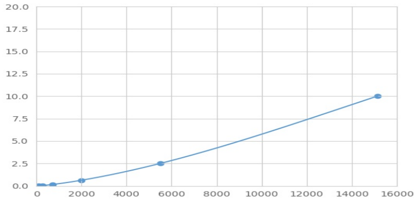
(一氧化氮合酶运输因子)检测试剂盒标准曲线
