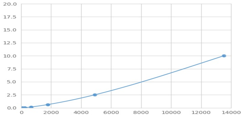
(血小板衍生生长因子AA)检测试剂盒标准曲线
