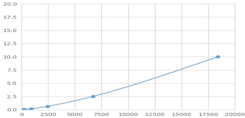
(血小板衍生生长因子受体β)检测试剂盒标准曲线
