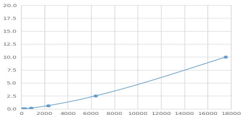
(脯氨酸/丝氨酸丰富卷曲螺旋蛋白1)检测试剂盒标准曲线
