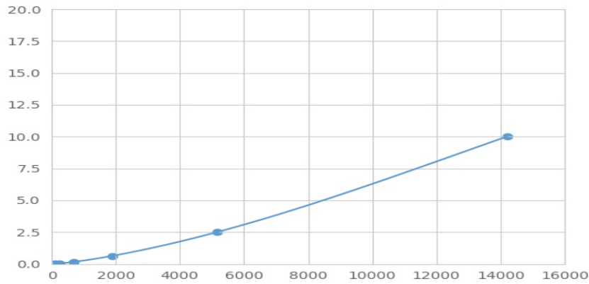
(Mg 2+ /Mn 2+ 依赖性蛋白磷酸酶1D)检测试剂盒标准曲线
