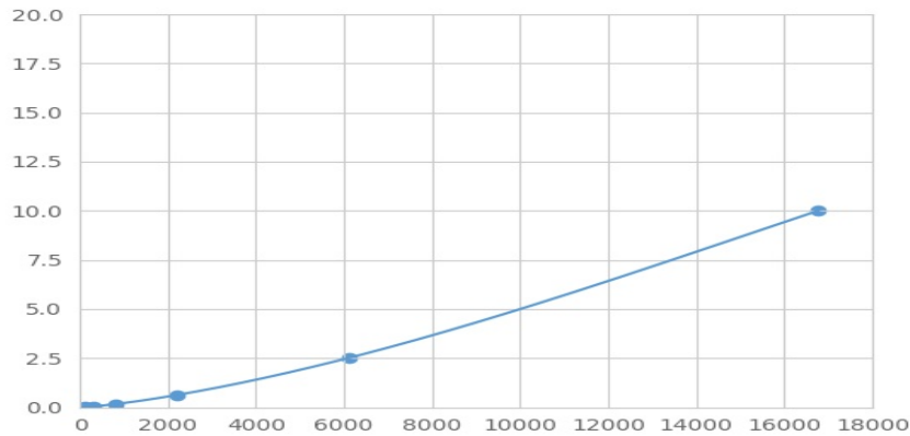
(蛋白酪氨酸磷酸酶受体Z)检测试剂盒标准曲线
