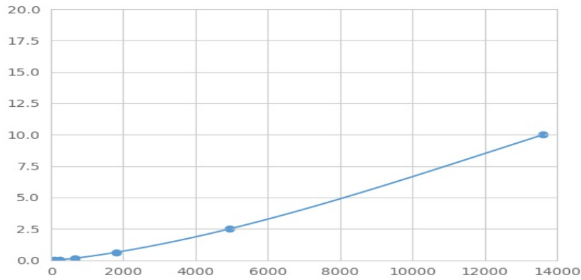
(视黄醇结合蛋白1)检测试剂盒标准曲线
