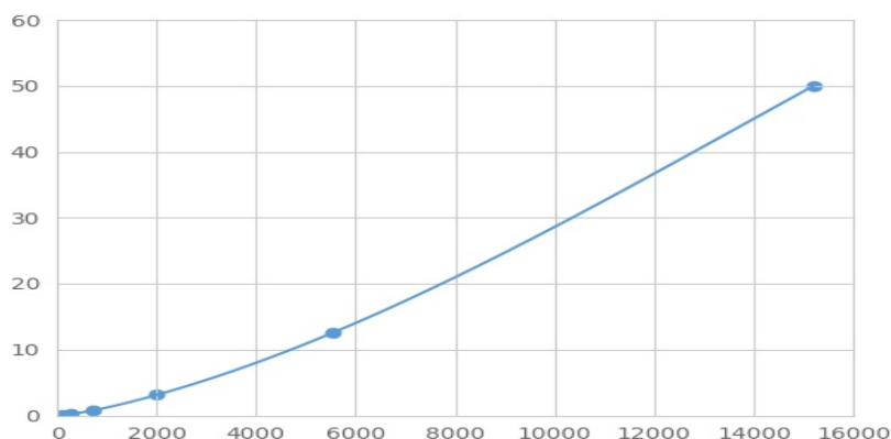
(肌糖 \delta ) 检测试剂盒标准曲线
