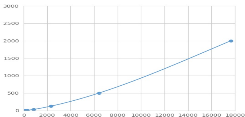
(分层蛋白)检测试剂盒标准曲线
