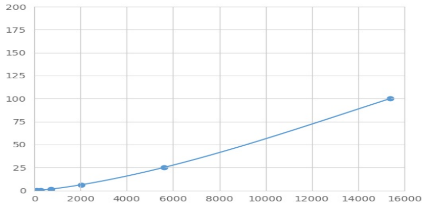
(转酮醇酶)检测试剂盒标准曲线
