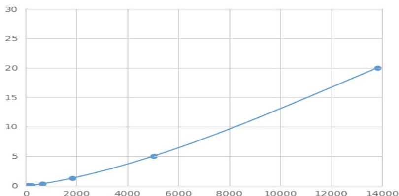
(泛素特异性肽酶14)检测试剂盒标准曲线
