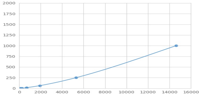
(血管内皮生长因子165)检测试剂盒标准曲线
