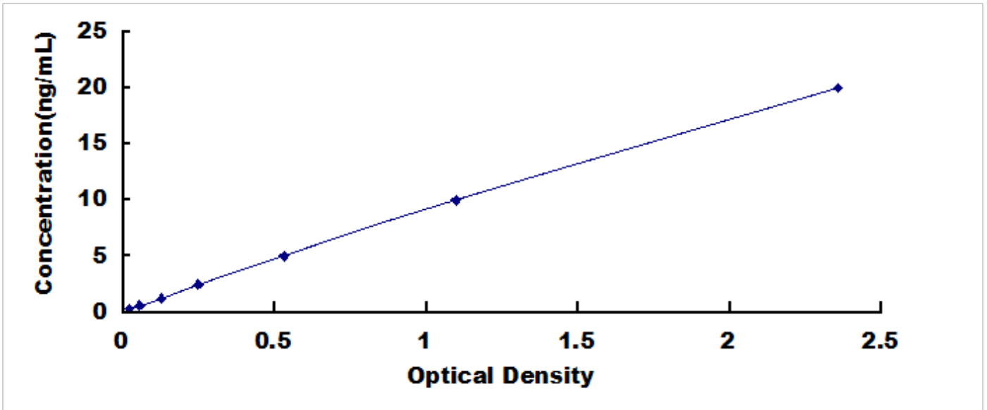
小鼠叉头框蛋白 P3 (FOXP3) 检测试剂盒标准曲线
