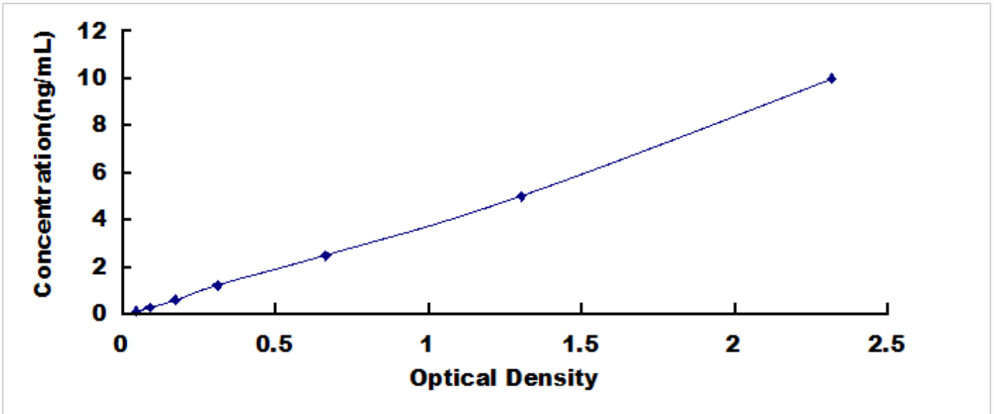
人基质金属蛋白酶 1 (MMP1) 检测试剂盒标准曲线
